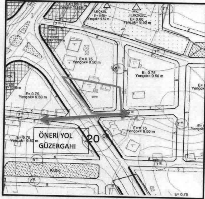
1/1000 ÖLÇEKLİ UYGULAMA İMAR PLANI (ÖNERİ)
